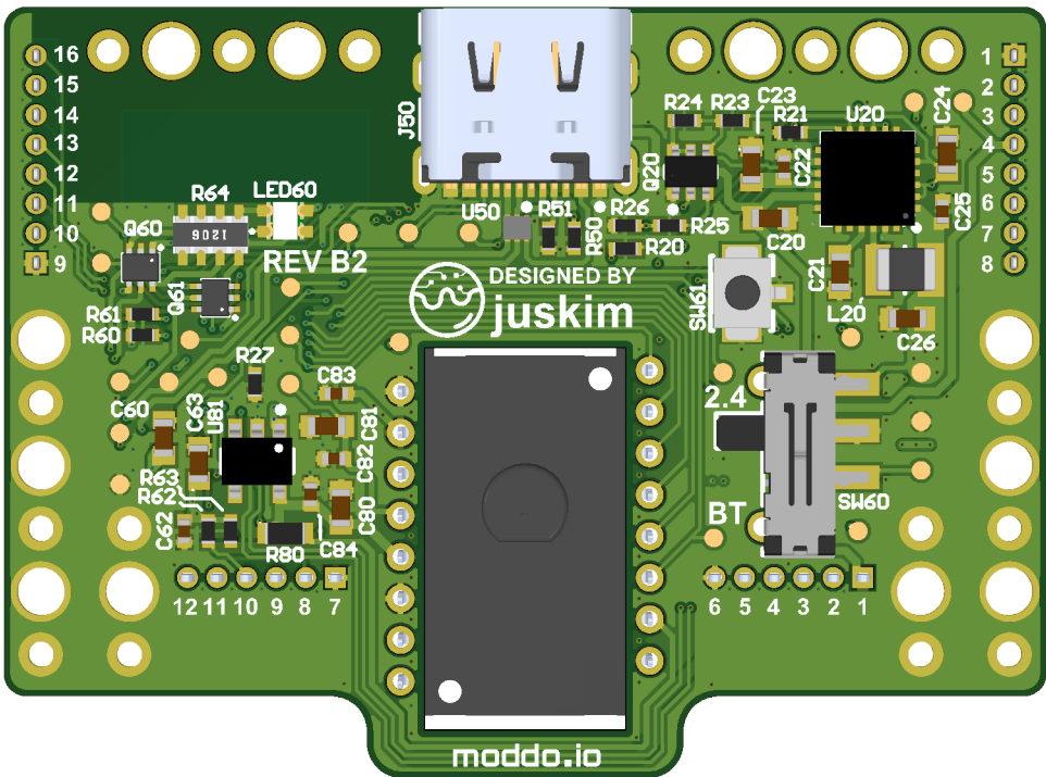
BOTTOM
