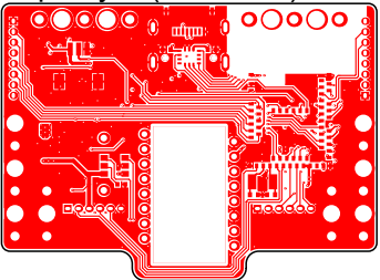
Top Layer (Scale 1:1)
