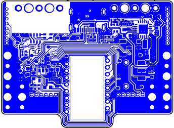
Bottom Layer (Scale 1:1)
